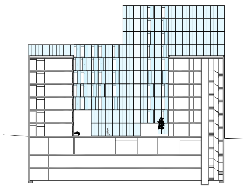
Seccion 3
