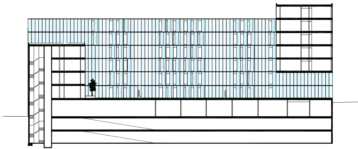
Seccion 1
